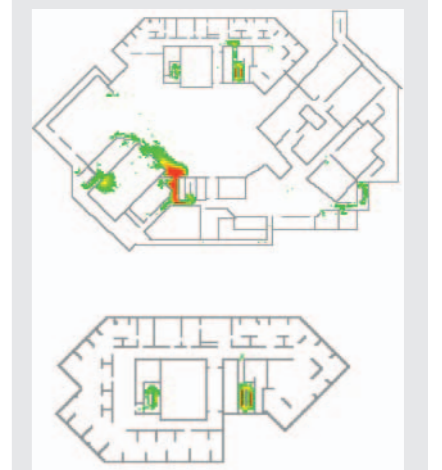
Evakuationssimulation
